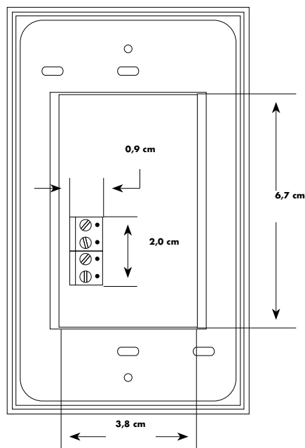
RÜCKANSICHT
