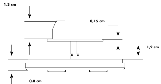
UNTERANSICHT
